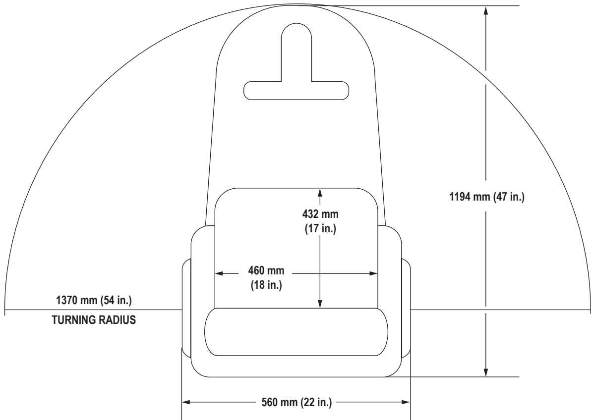
Colt Plus (SC710) Dimensions
